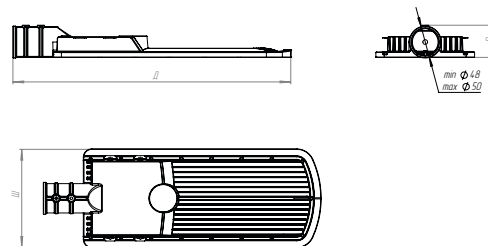
ГАБАРИТНЫЙ ЧЕРТЕЖ
