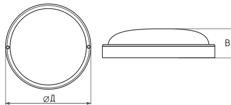
Диаметр, м: 0,140-0,200; Высота, м: 0,045
