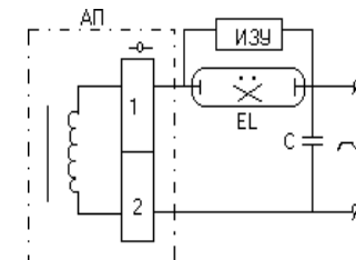
Рис.2 - Электрическая схема
